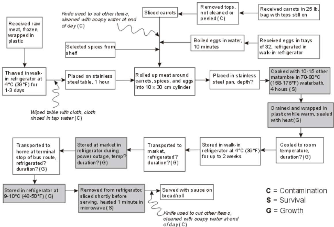
Figura 2. Diagrama de flujo para la preparación de matambre, Brote de Botulismo en Buenos Aires, enero de 1998.
